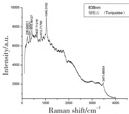
图3 闰楼ZMD-3拉曼图谱
